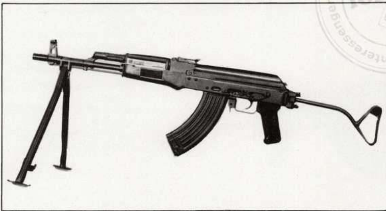
AKM-special assault rifle with bipod and metal butt AKM-Spezialsturmgewehr mit Zweibein und Metall- kolben Fusil d'assaut à vocation spéciale AKM avec bipied et crosse métallique Fusil de asalto especial AKM con bipode y culata metálica AKM-espingarda de assalto especial com bipé e coronha metálica ذات منصّب واخص معدني بندقية اقتحام خاصة AKM
