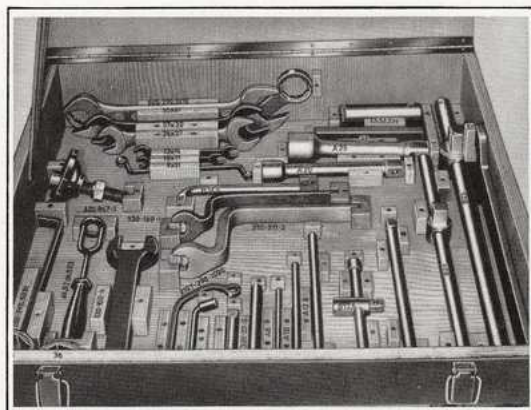
Tool sets for special vehicles Werkzeugsätze für Spezial- fahrzeuge Lot d'instrument pour véhicu- les spéciaux Juegos de herramientas para vehículos especiales Jogos de ferramentas para viaturas especiais مجموعة الآلات لل عربات الخاصة
